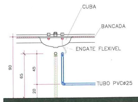
VISTA FRONTAL DA LIGAÇÃO DE ÁGUA/ESGOTO
