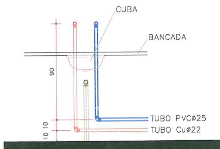
VISTA LATERAL DA LIGAÇÃO DE ÁGUA/ESGOTO Sem Escala
