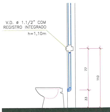
VISTA FRONTAL DA LIGAÇÃO DE ÁGUA/ESGOTO Sem Escala
